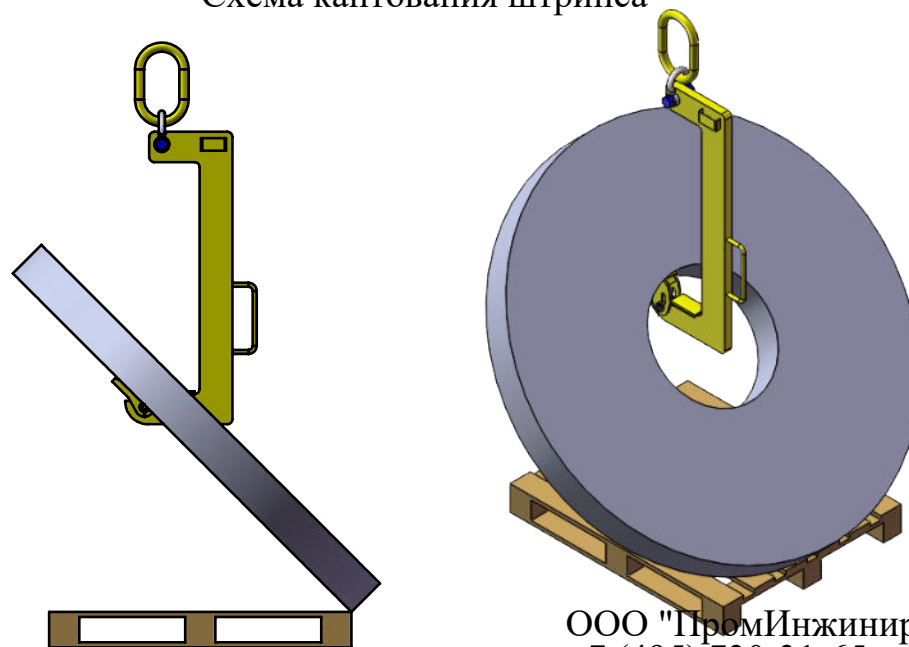
Схема кантования штрипса
